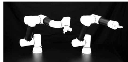
慶應義塾大学と共同で開発したロボットアーム「ハプティクスプラットフォーム」 【株式会社小野電機製作所】
